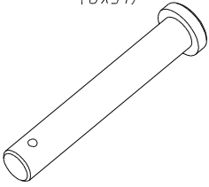
Палец С52.00.00.24 (8x51)
