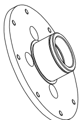
Фланец ТН190.03.001 (до 01.02.2015, Ø 178, в отв. М8)
