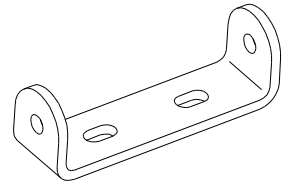
Пластина С52.00.00.35
