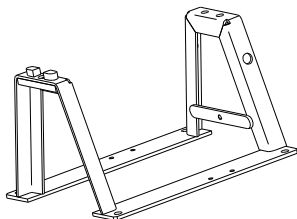
Опора С52.30.00.00
