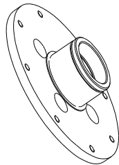
Фланец ТН190.03.001 ( \Phi 160, 6 отв. М8)
