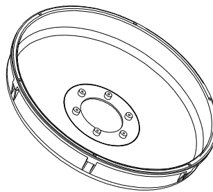
Крышка ТН190.03.002
