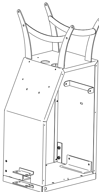
Корпус ТН190.08.000
