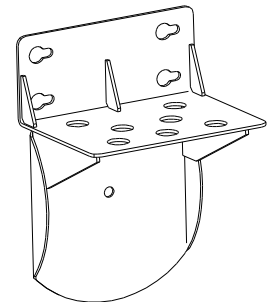
Якорь ТН190.04.000
