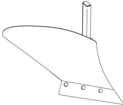
Окучник С52.150.70.00
