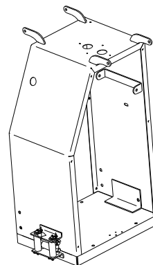
Корпус С52.10.00.00 (до 01.09.2013)
